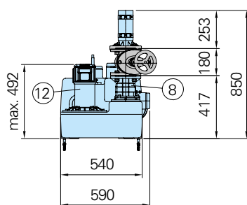
PVC-Zulaufschieber DN 100
