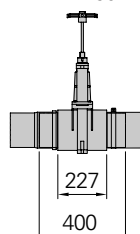
PVC-Zulaufschieber DN 150
